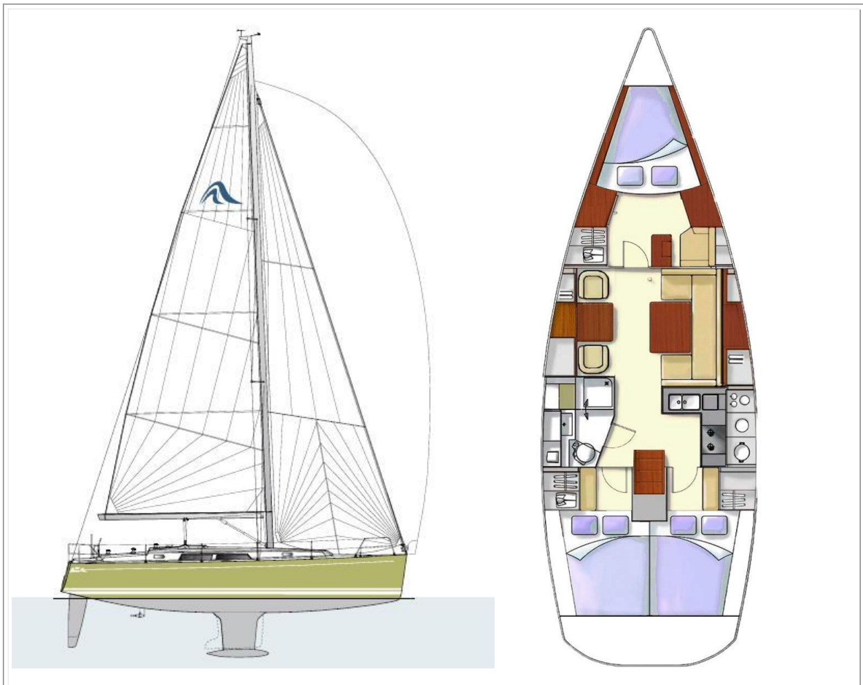
SEITENANSICHT & GRUNDRISS
